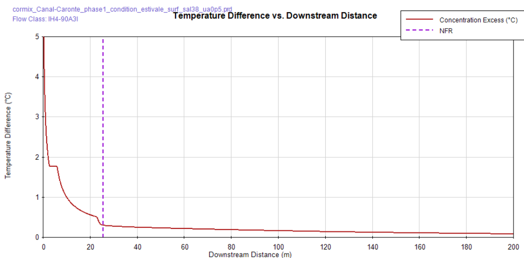
Figure 3-4 : Ecart de température du panache par rapport au milieu ambiant en fonction de la distance au point de rejet pour une salinité en surface à 32.5 ppt (haut), à 36.5 ppt (milieu) et à 38 ppt (bas).
