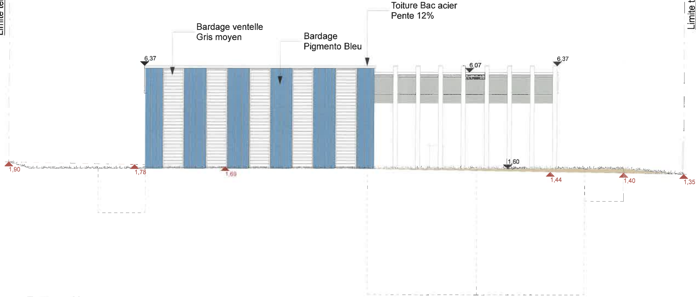
Façade Nord
